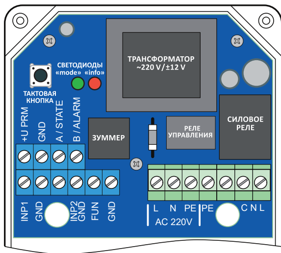
Рис. 1. Плата блока управления GIDROLOCK STANDARD RADIO
