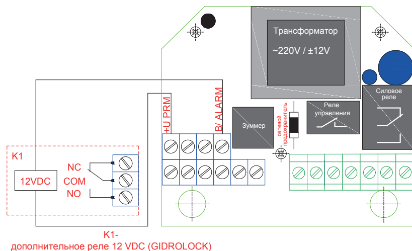
Рис. 6. Схема подключения дополнительного реле
