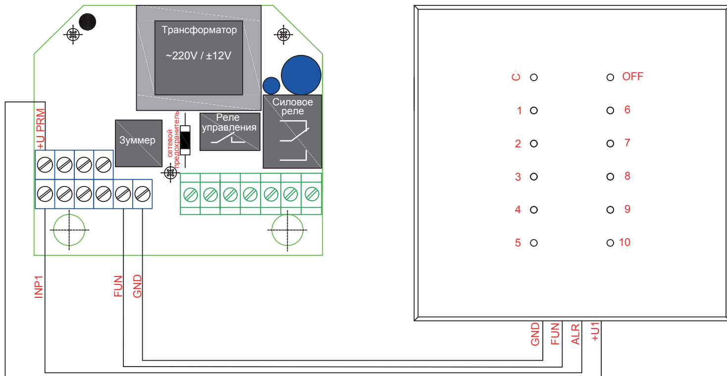
Рис. 8. Схема подключения выносного радиоприемника системы GIDROLOCK RADIO
