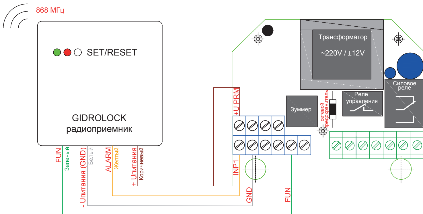
Рис. 10. Схема подключения выносного блока радиоприемника S32
