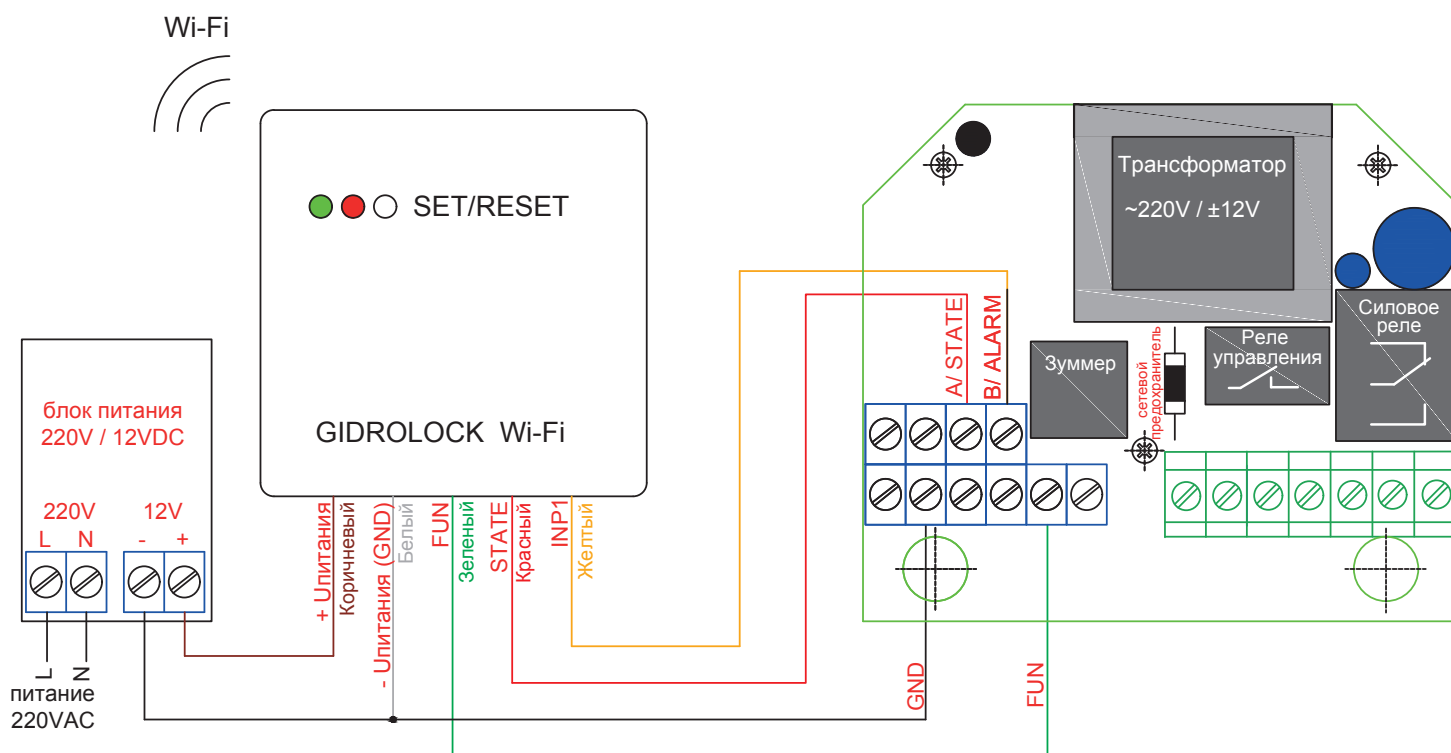
Рис. 11. Схема подключения модуля Wi-Fi GIDROLOCK к блоку питания 12 В
