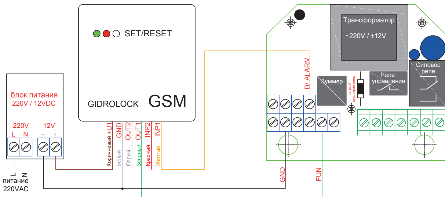
Рис. 9. Схема подключения GSM- модема GIDROLOCK с внешним блоком питания 12 В
